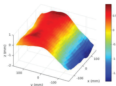
FIGURE 10 – Triangulation de la plaque au repos.
