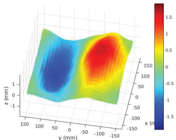
FIGURE 16 – Déformée de la plaque identifiée à 160 Hz.
