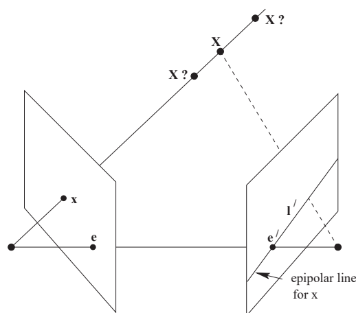
FIGURE 1 – Principe de la triangulation, tiré de [14].
