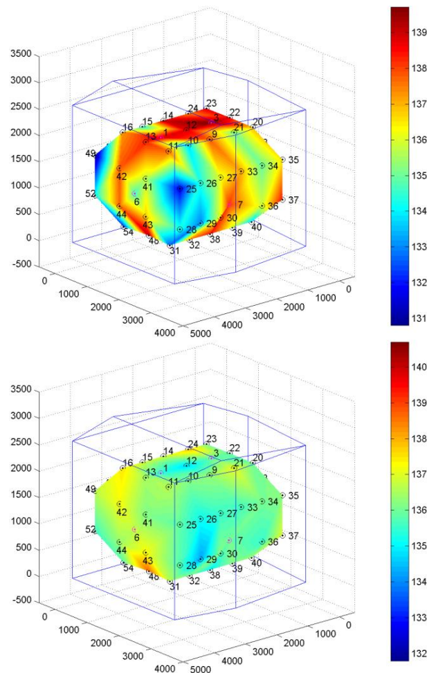
FIGURE 8 – Niveau acoustique relevé sur les microphones en moyenne sur l’octave 250Hz
