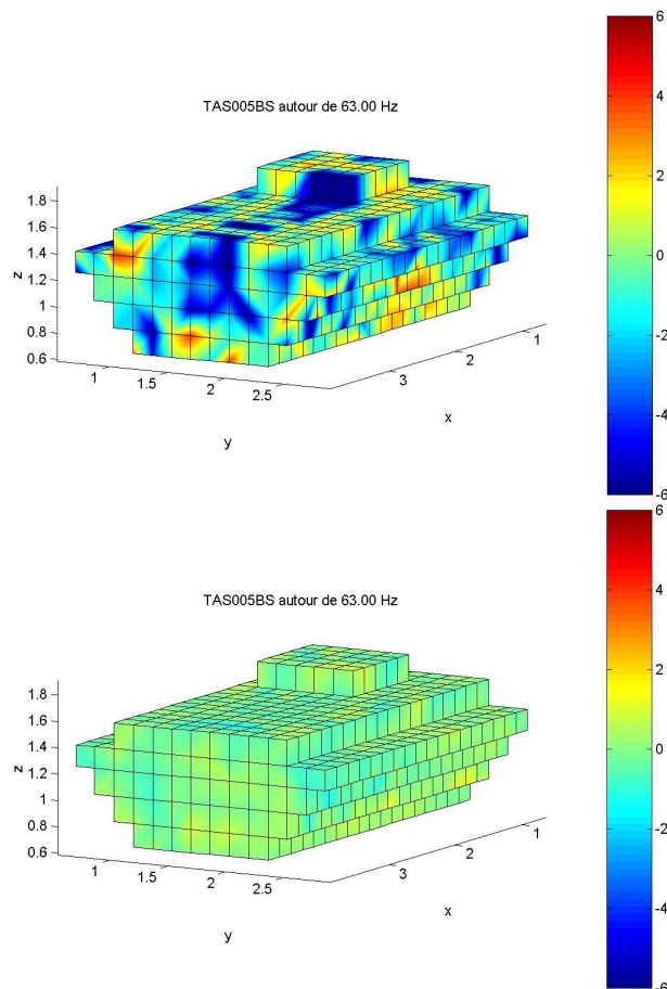
FIGURE 4 – Champ acoustique résultant sur le satellite : sans (h) et avec (b) égalisation de l'octave 63Hz
