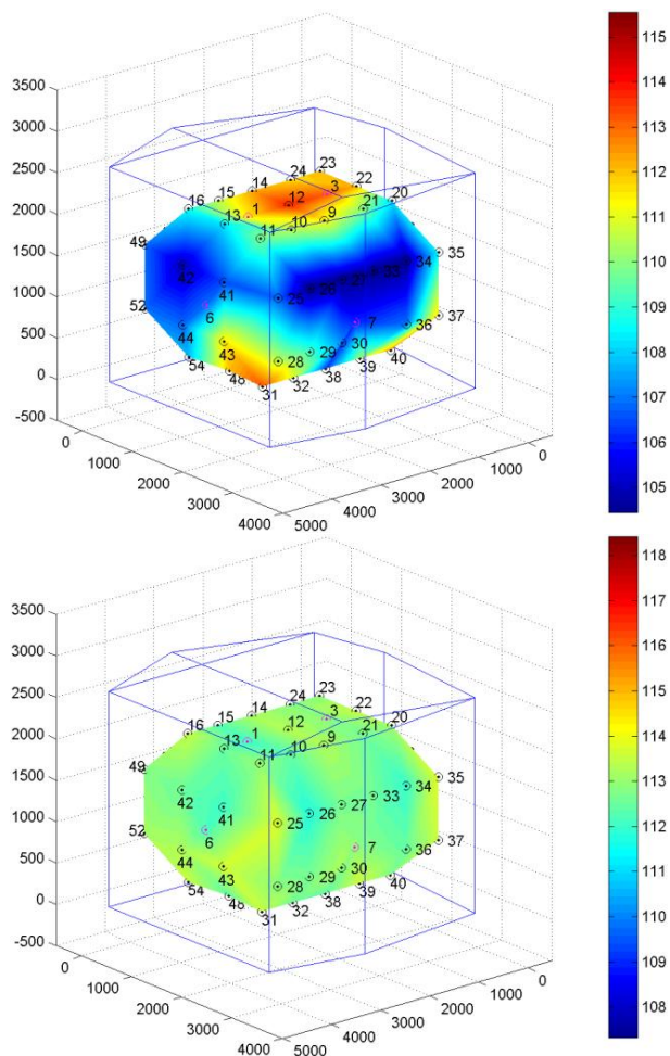
FIGURE 7 – Niveau acoustique relevé sur les microphones en moyenne sur l’octave 63Hz
