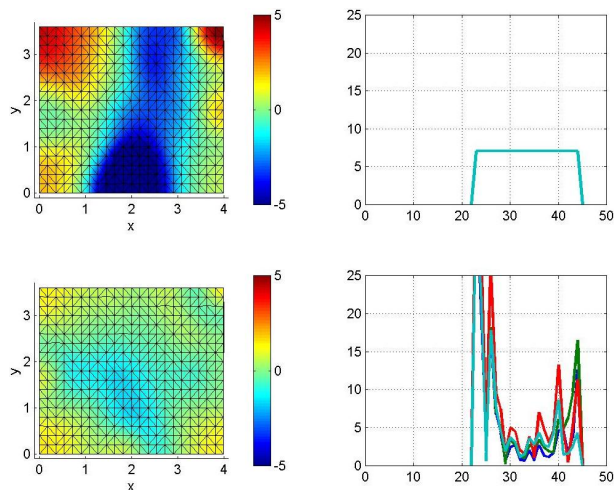
FIGURE 3 – Principe de l'égalisation BF
