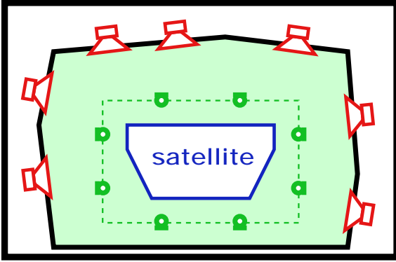
FIGURE 2 – Schéma de principe de l'installation
