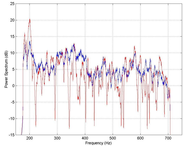
FIGURE 6 – Somme de 8 sources aux "MF" : 1 signal commun (rouge) ou 8 signaux décorrélés (bleu)
