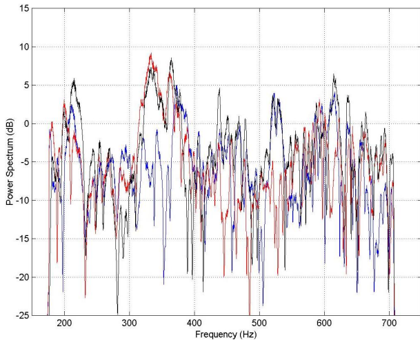
FIGURE 5 – Somme de 2 sources aux "MF" : S1 seule (rouge), S2 seule (bleu) et somme (noir)
